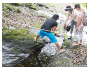
ポットホール散策
