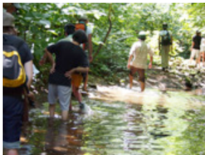
三原山を登る 澄み切った滝壺でひと泳ぎ
